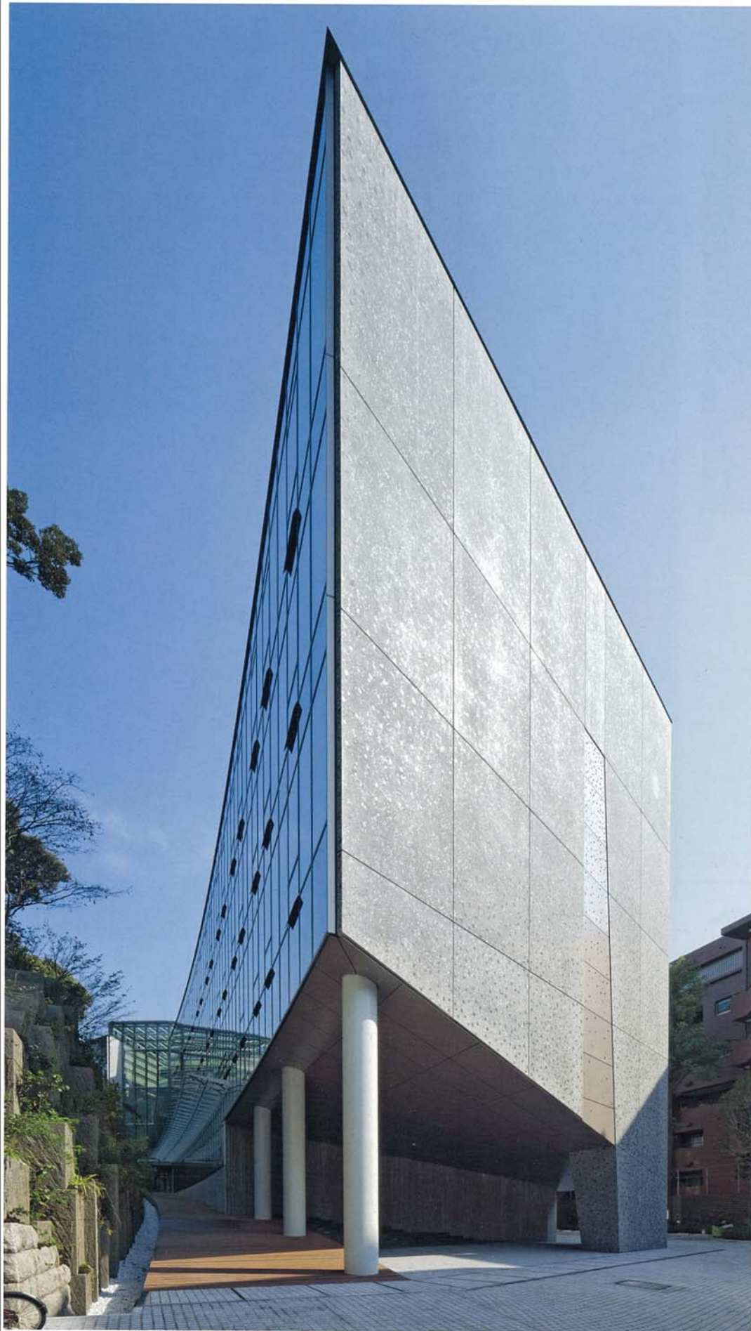
アプローチスロープより事務所棟を見る。長手は森に面して緩やかにカーブするカーテンウォール。短手は花崗岩と石灰岩の砕石を打ち込んだPCa版
